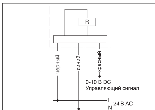
Схема подключения
