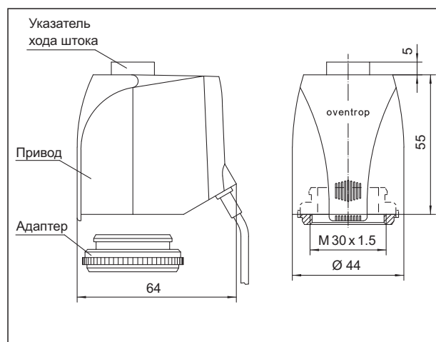
Размеры
